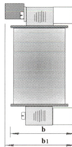
Zijaanzicht
