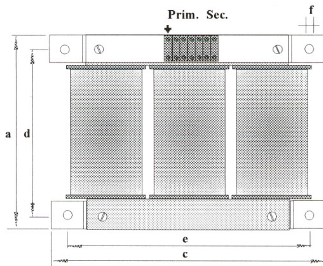
Vooraanzicht
