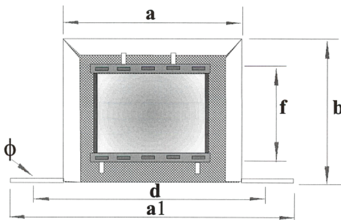
Vooraanzicht
