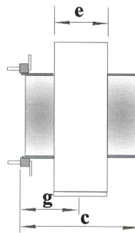
Zijaanzicht
