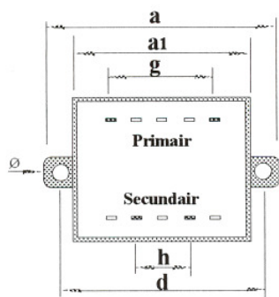
EI 42/14 - EI 48
