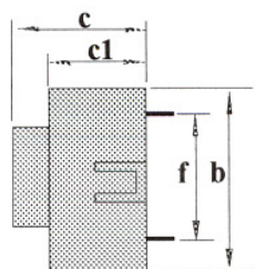
EI 42/14 - EI 48
